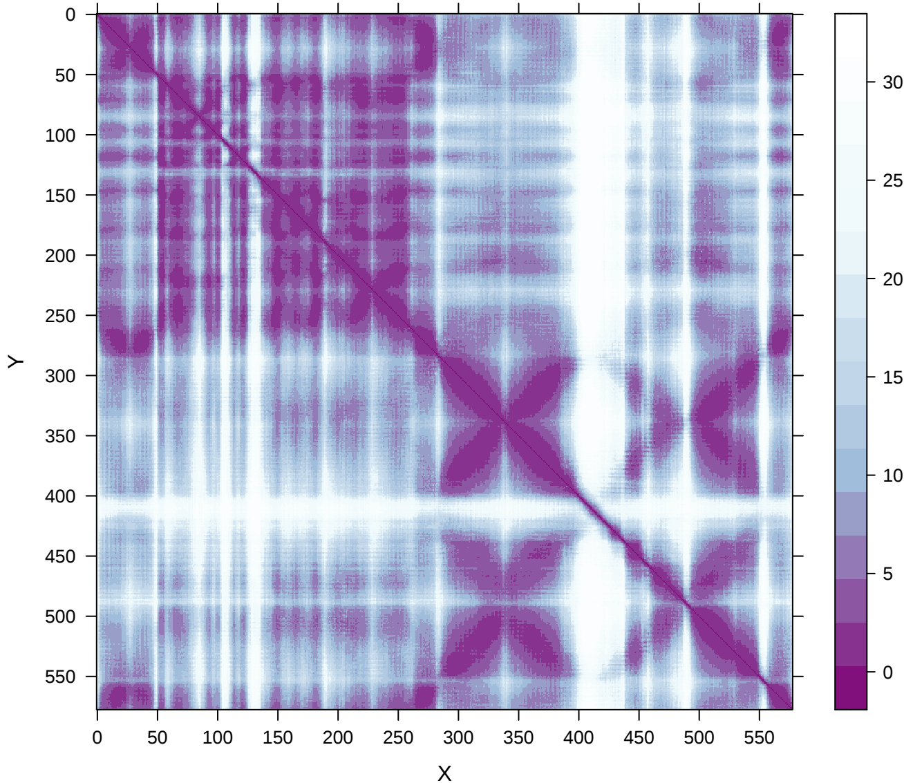
PAE | Eleos.Eleos__LeoA.0.V-plddts_80.93074
