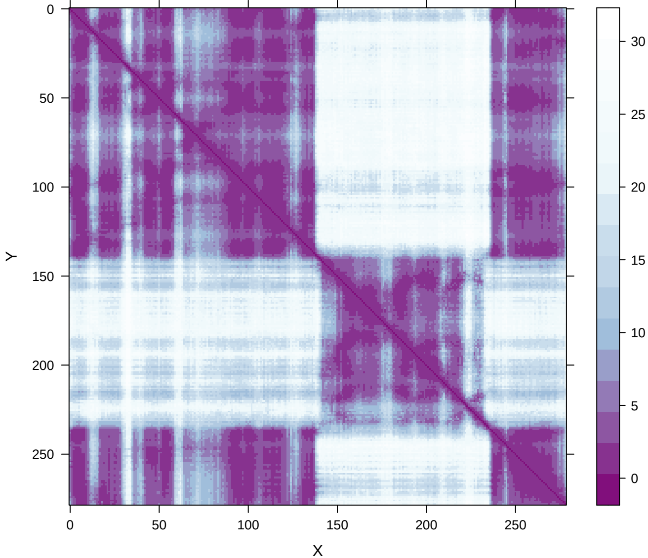
PAE | RexAB.RexAB_RexA.0.V-plddts_85.0085
