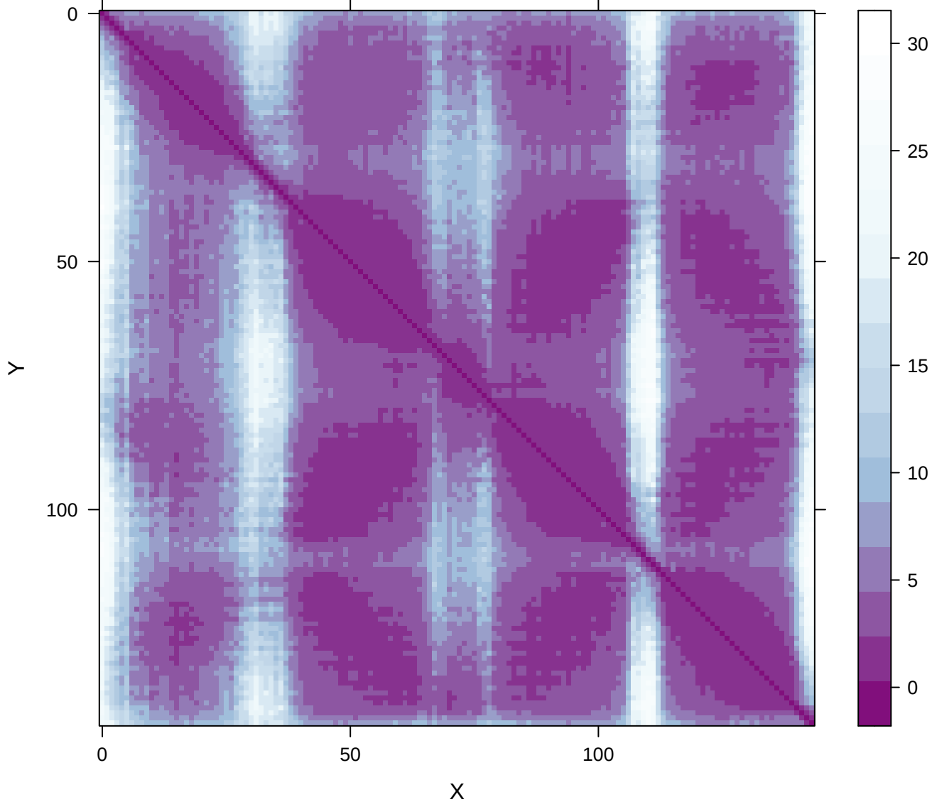
PAE | RexAB.RexAB_RexB.0.V-plddts_86.87723
