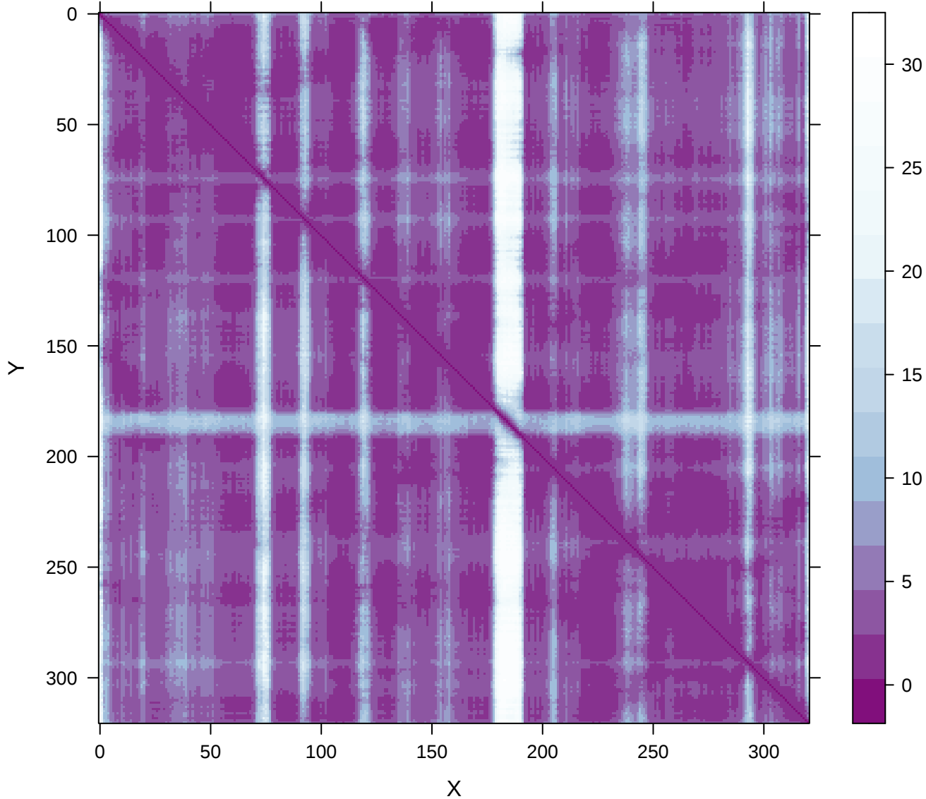
PAE | SspBCDE.SspBCDE__SspB.0.V-plddts_92.22861
