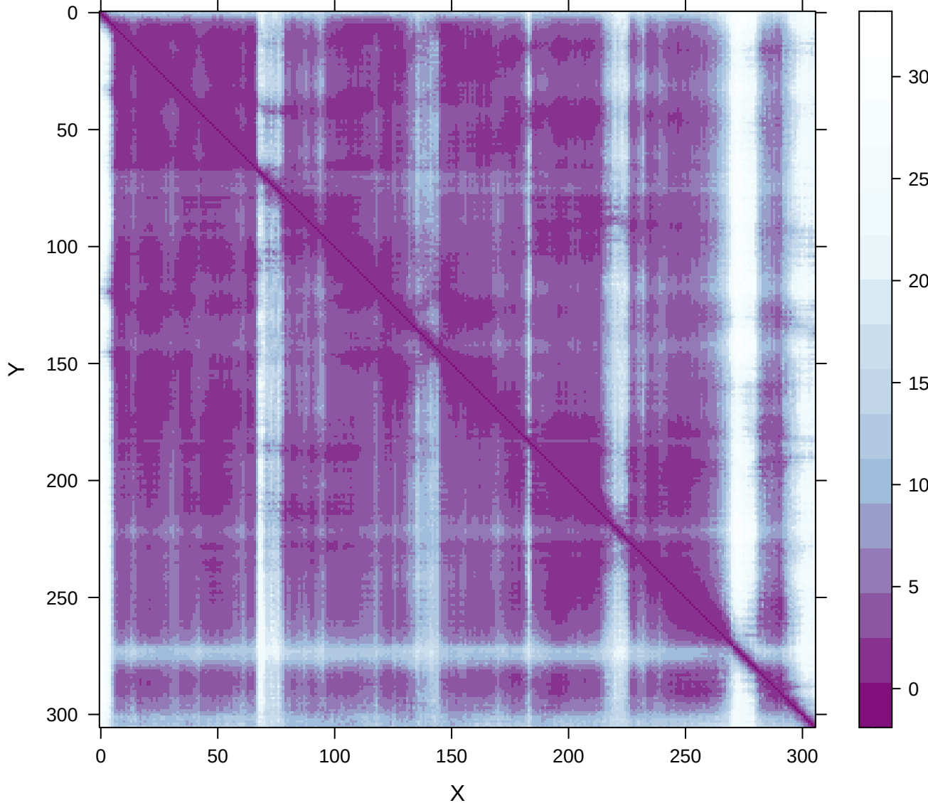
PAE | SspBCDE.SspBCDE__SspD.0.V-plddts_86.98506
