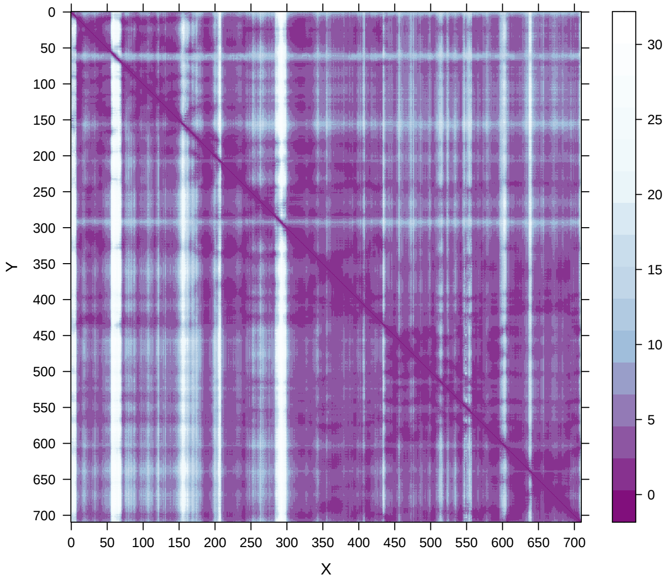
PAE | Borvo__BovA-plddts_90.79263
