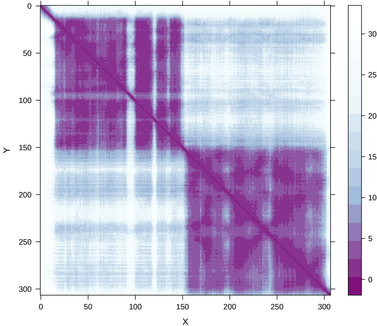
PAE | BstA__BstA-plddts_84.76542
