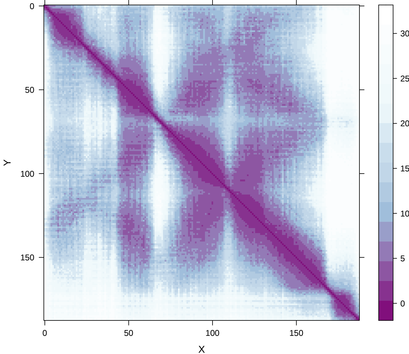
PAE | FS_HsdR_like_HP-plddts_74.75219
