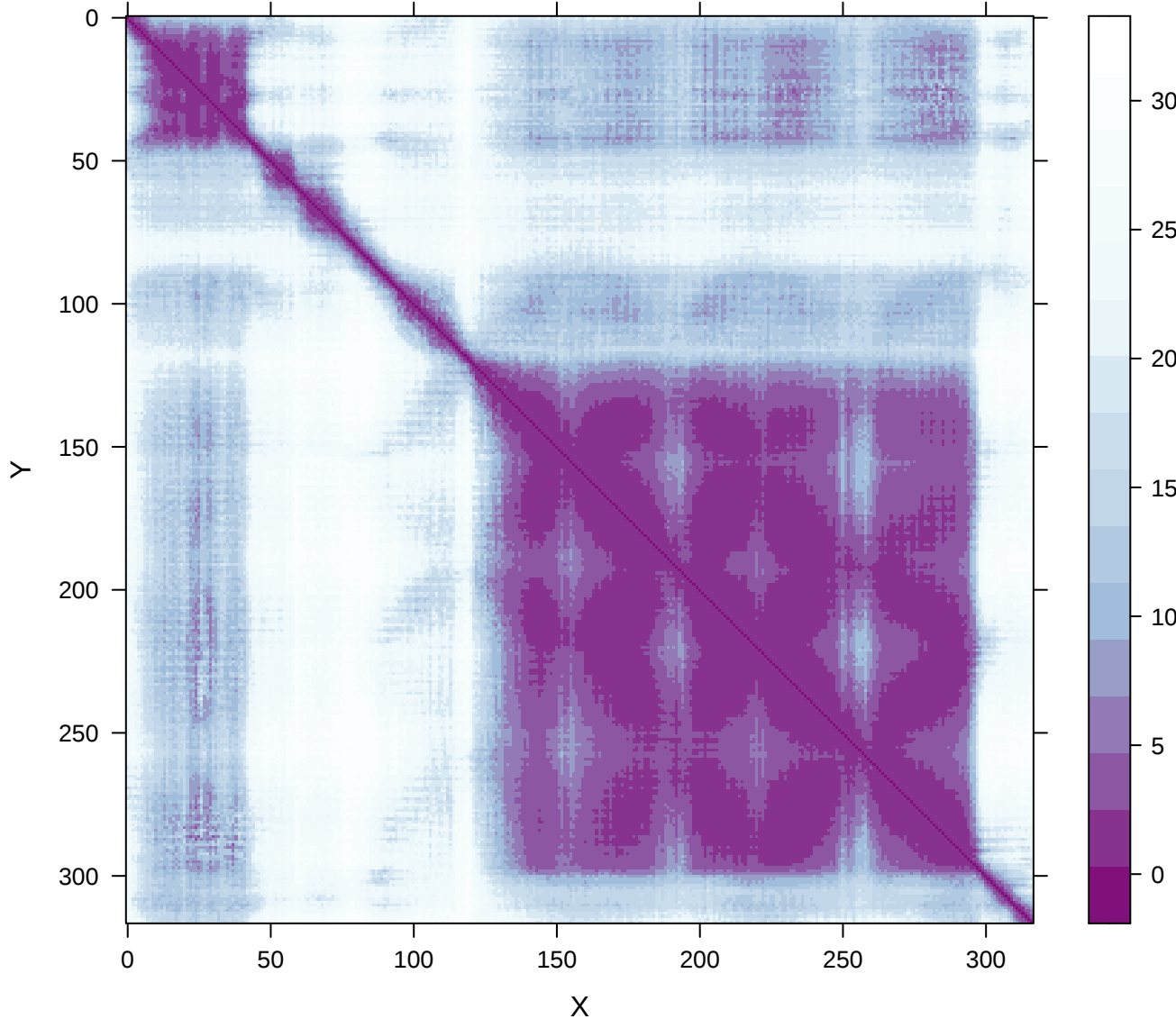
PAE | JukAB__JukB-plddts_67.28863
