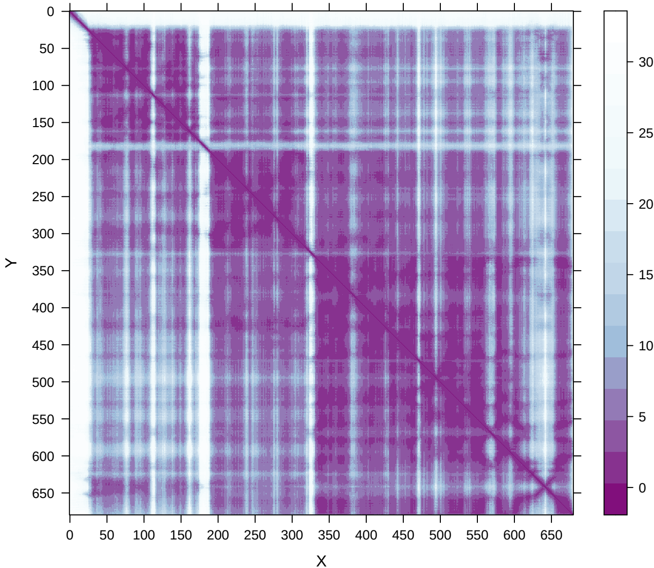
PAE | MADS__mad2-plddts_87.54253
