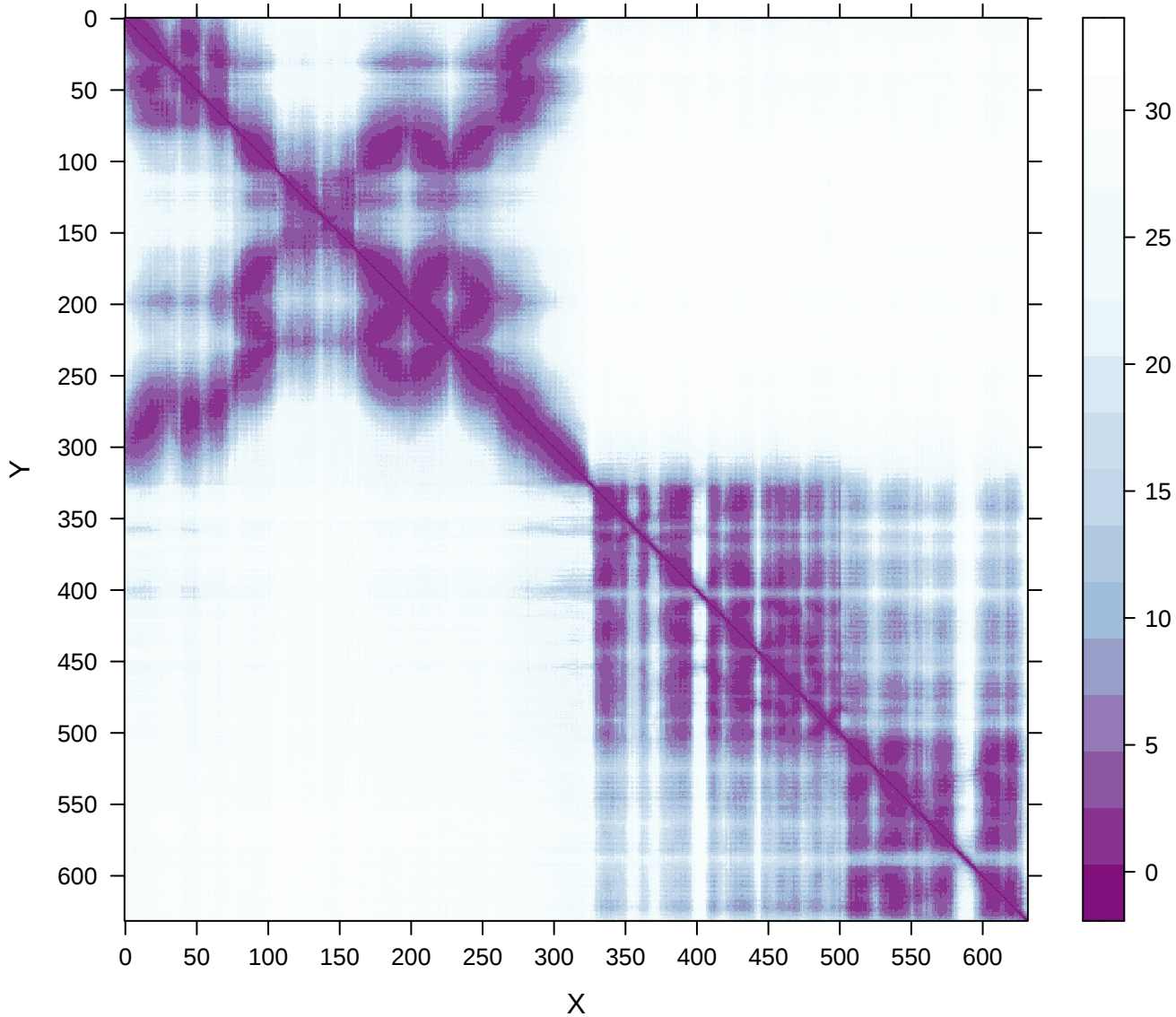
PAE | RloC__RloC-plddts_86.73175
