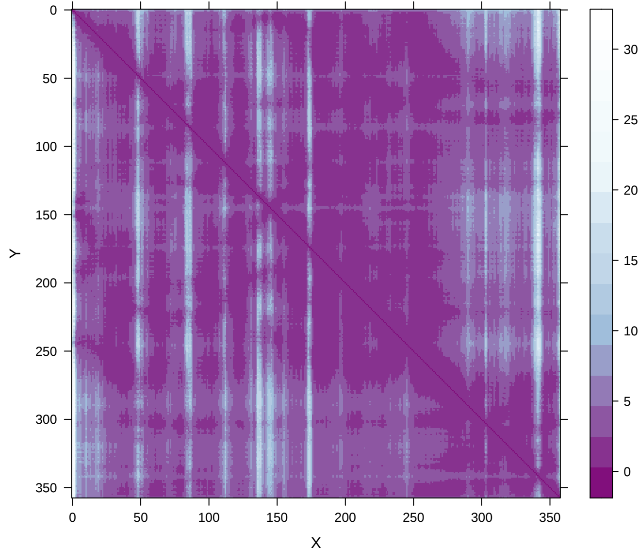
PAE | SoFic__SoFic-plddts_95.70819
