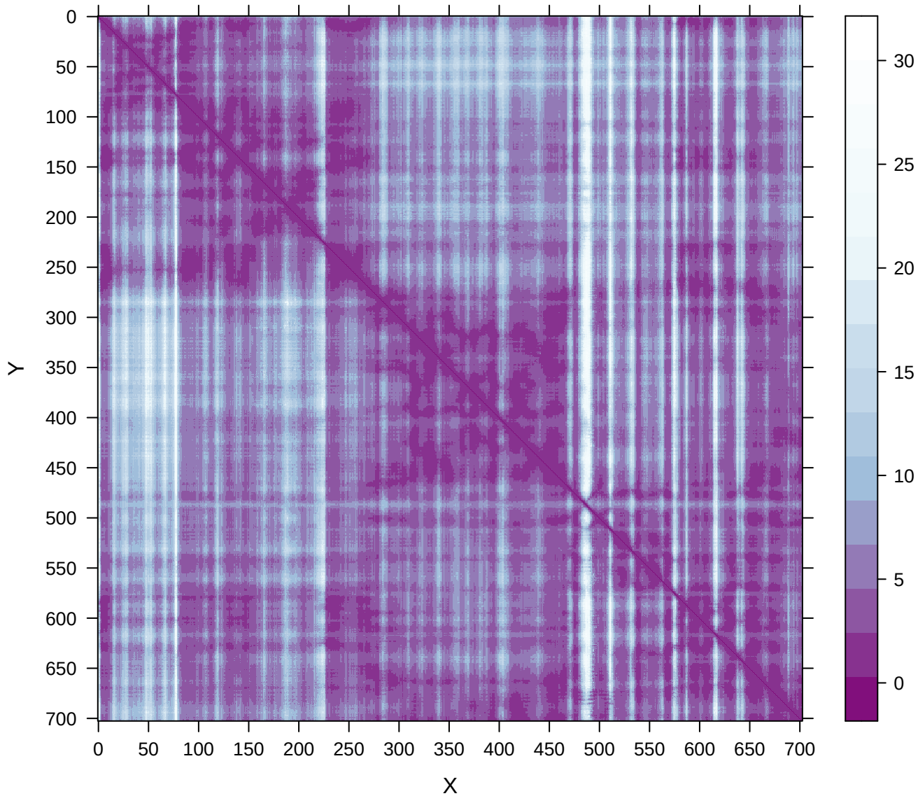
PAE | pAgo_pAgo_LongB-plddts_92.47739
